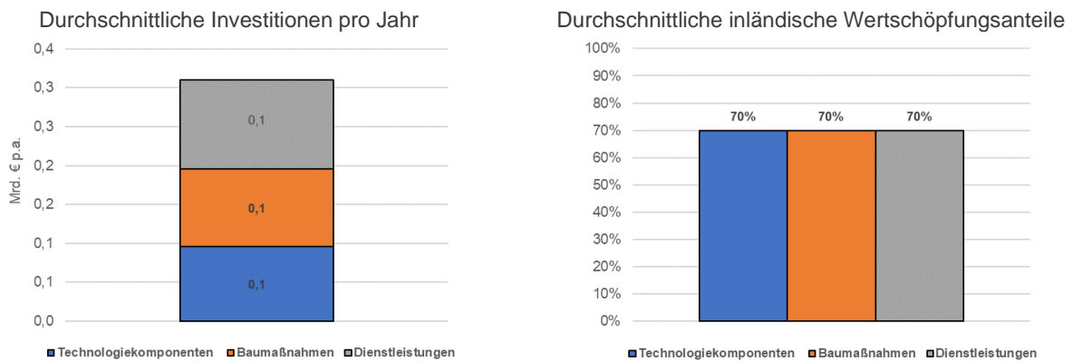
Abbildung 25: Investitionen und deren inländischer Wertschöpfungsanteil im Rahmen des Ausbaus von Solarthermie, 2020 – 2030
